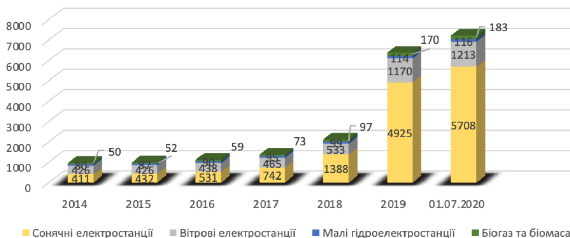
Встановлена потужність об'єктів відновлюваної енергетики, 2014 - 2020рр., МВт джерело: НКРЕКП
