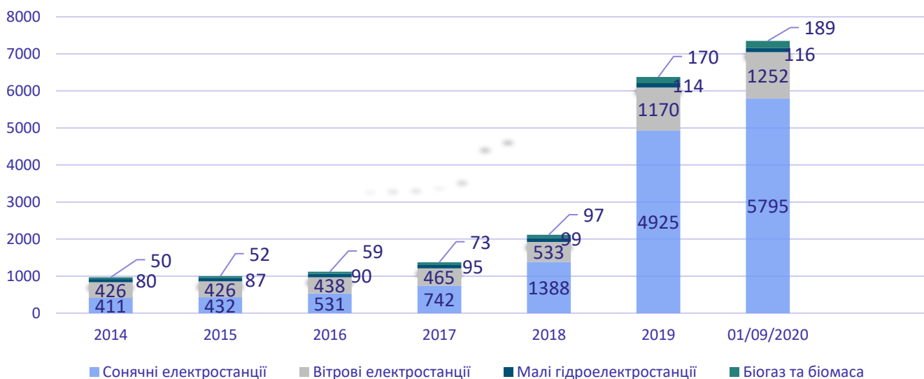
Встановлена потужність об'єктів відновлюваної енергетики, 2014 - 2020, МВт джерело: НКРЕКП
